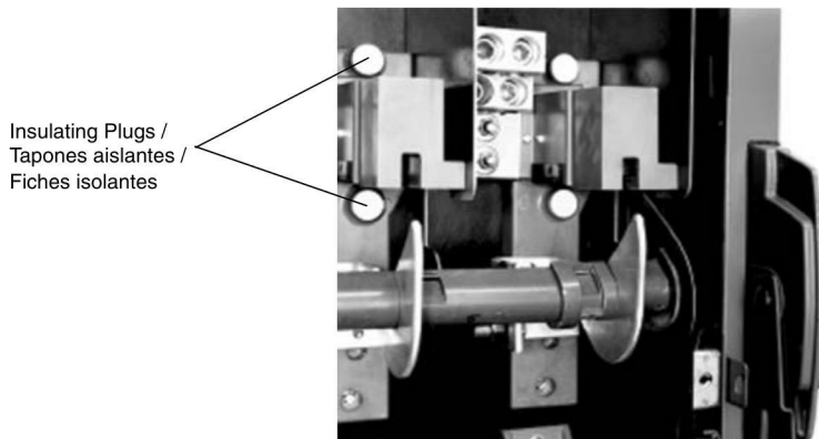
FIG. 2 : Pole Unit / Polo individual / Pôle individuel
